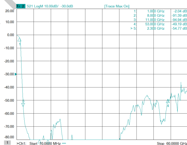
LIF-1G-001B型低通滤波器低温 (<5K) 典型测试曲线
