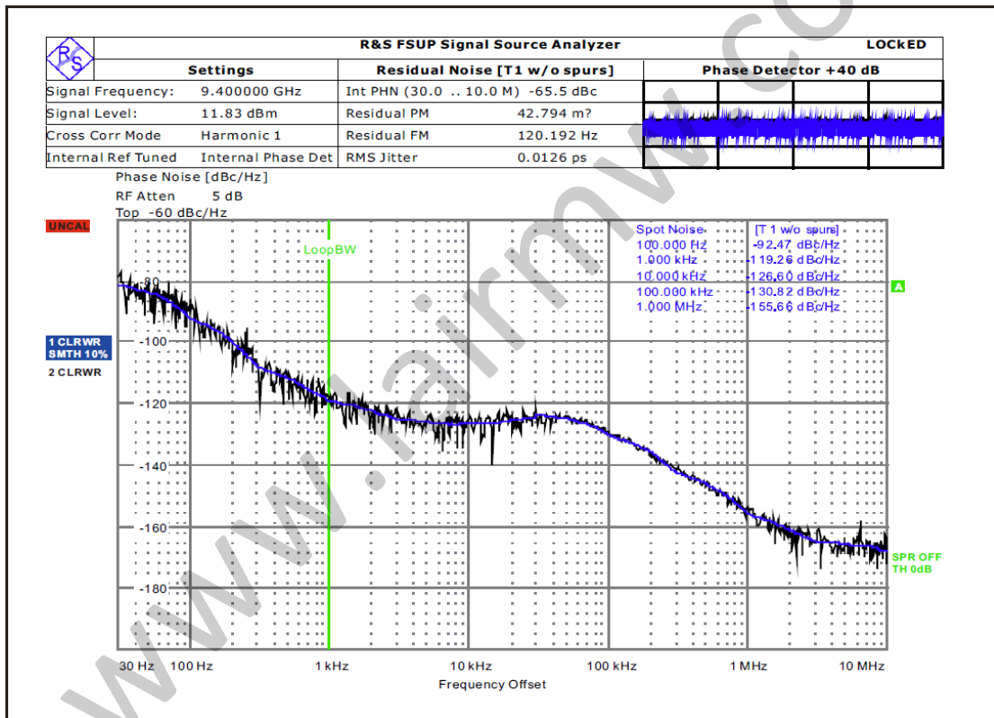
10GHz 相位噪声测试曲线 Phase Noise Curve
