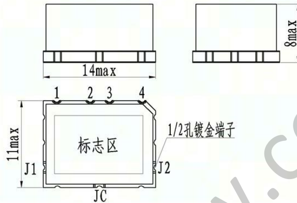
图 1 外形尺寸
