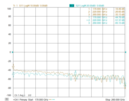
隔离度
