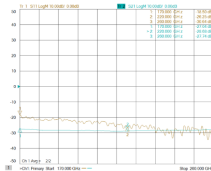
耦合度
