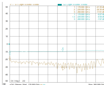
耦合度
