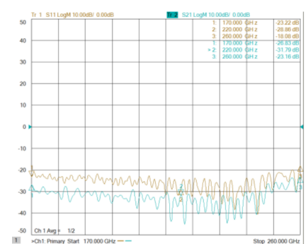
隔离度
